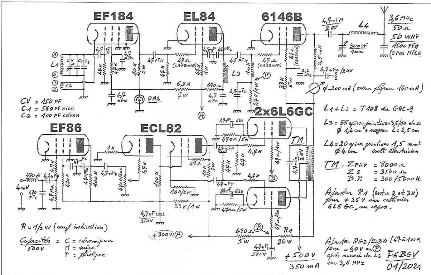
Schéma du BGV-80 bis
