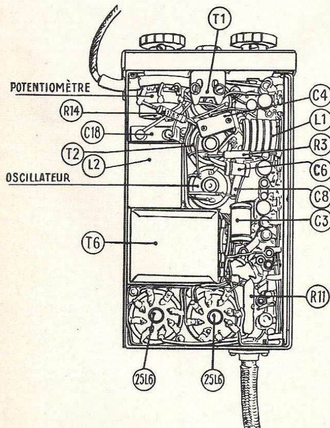
FIG. 3. — Disposition des éléments sous le chassis
